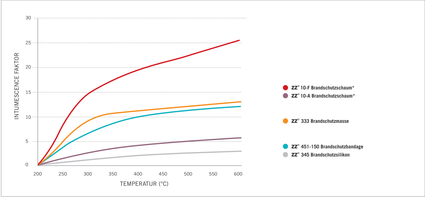
Intumeszenzvergleich der oben benannten Baustoffe
